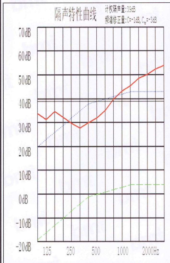
1/3 倍频程中心频率隔声特性曲线
